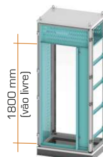
Com porta inteira IP 43/IP 54 E IP 65. Uso com espelhos interno
