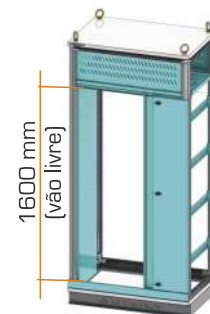
Com portas segmentadas IP 43/54.
