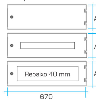
Espelhos articuláveis
