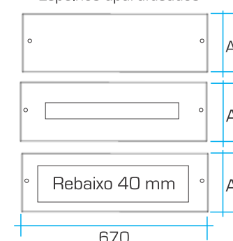
Espelhos aparafusados
