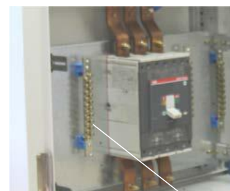
Placa de Montagem
