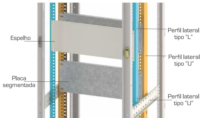
Placa de montagem segmentada e espelho interno fixada diretamente nos perfis verticais
